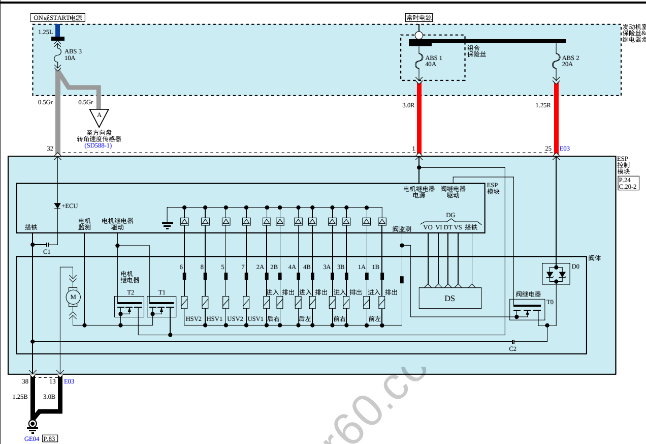
电控稳定程序(ESP)系统(4)
